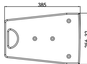
侧视图
