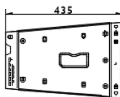
侧视图
