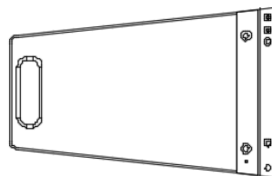
侧视图
