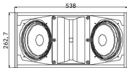
主视图
